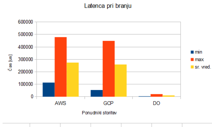
Slika 1.12: Minimalna, maksimalna in povprečna latenca pri branju enega bloka.
