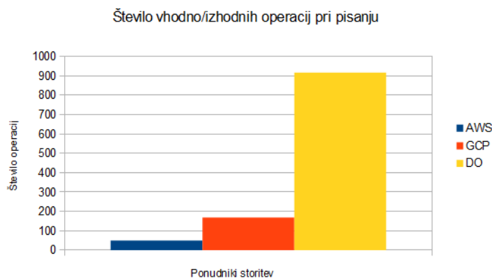
Slika 1.15: Število vhodno/izhodnih operacij pri pisanju.
