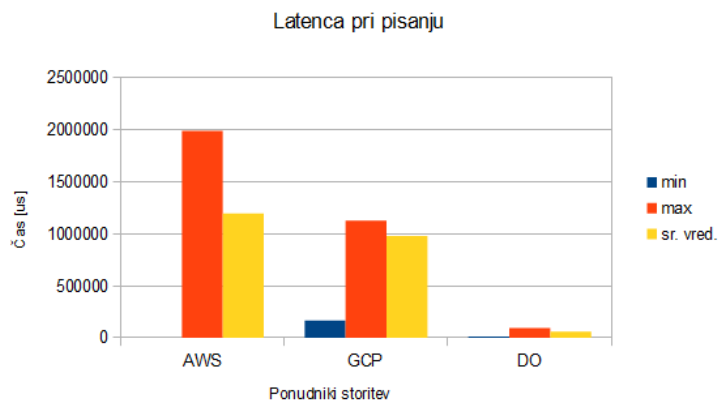
Slika 1.13: Minimalna, maksimalna in povprečna latenca pri pisanju enega bloka.
