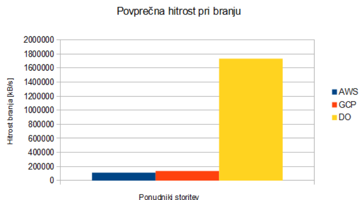
Slika 1.8: Povprečna hitrost pri branju.
