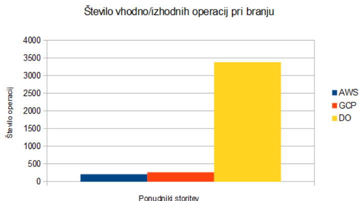
Slika 1.14: Število vhodno/izhodnih operacij pri branju.
